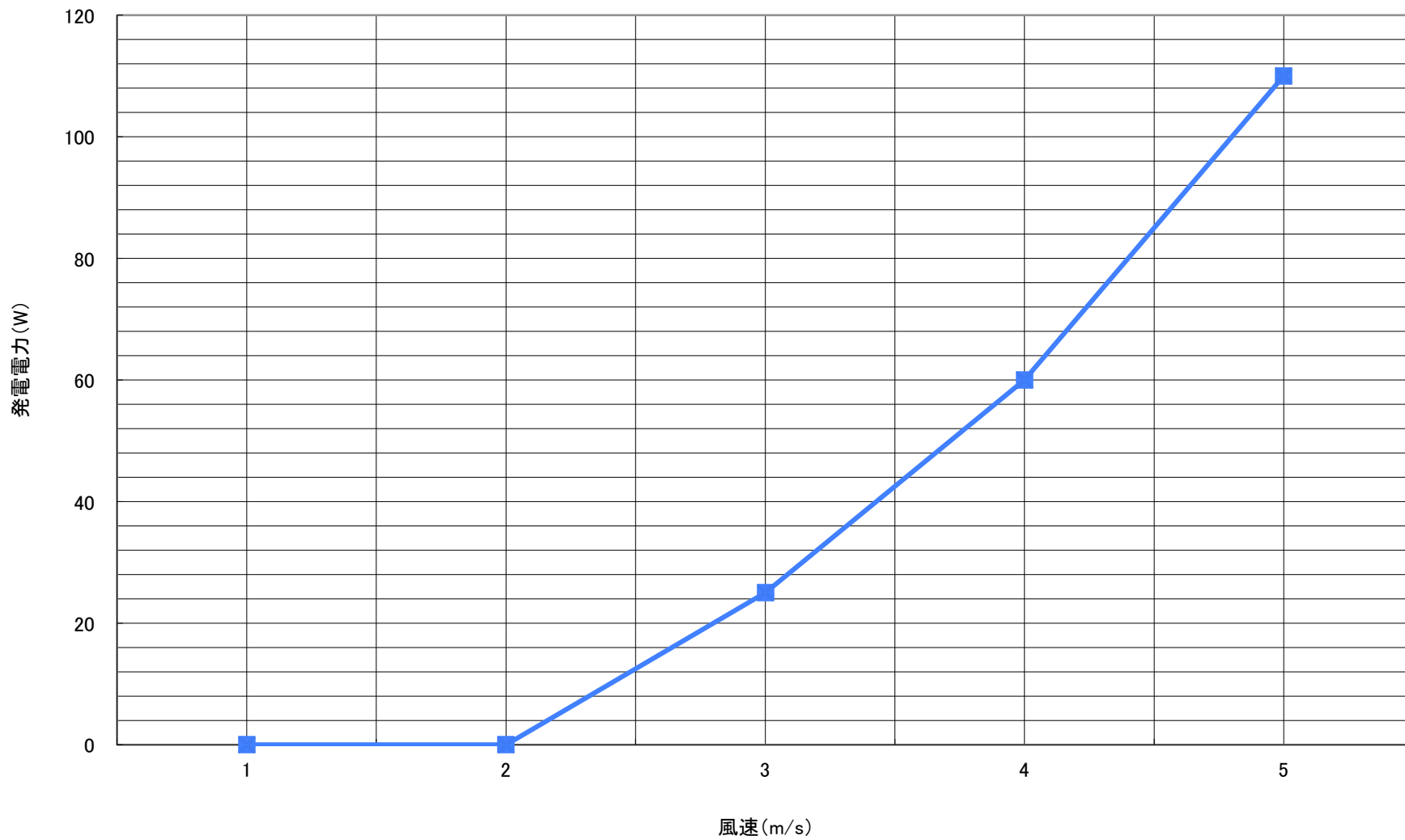
AD-1500PRO 風速(低風速) vs 発電電力(1~5m/s)
